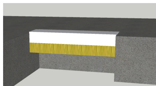
50 mm FireFree® B280 Brandgips støbt på 50 mm FireFree® Støbeplade
